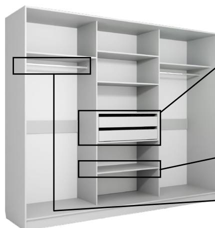
Конструкция 3-х дверного шкафа-купе Виват
